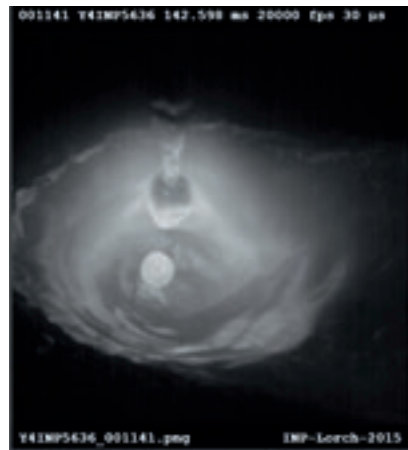
Der Primärtropfen bildet sich am Drahtende.
